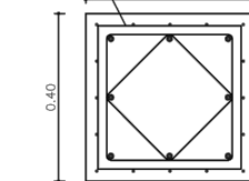
ALÇAT A1_E 1:25 A3_E 1:50 SECCIÓ A1_E 1:10 A3_E 1:20
