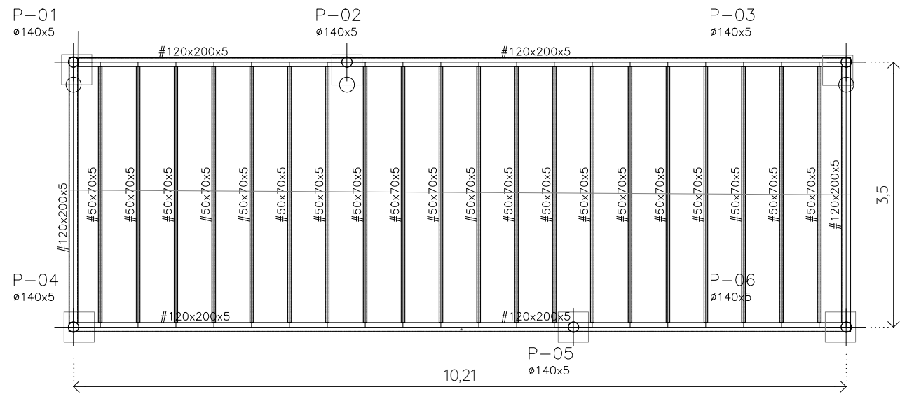
Planta Estructura
