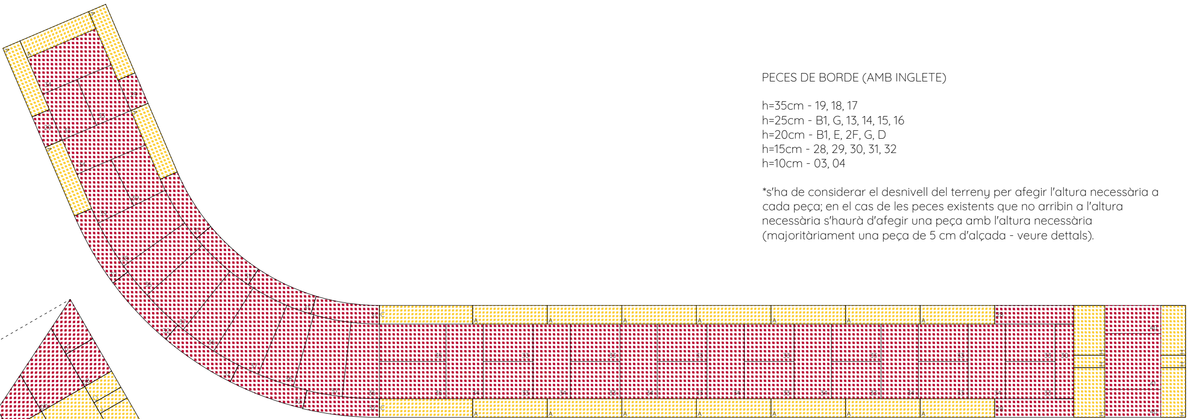
PLANTA E02 - 1/30
