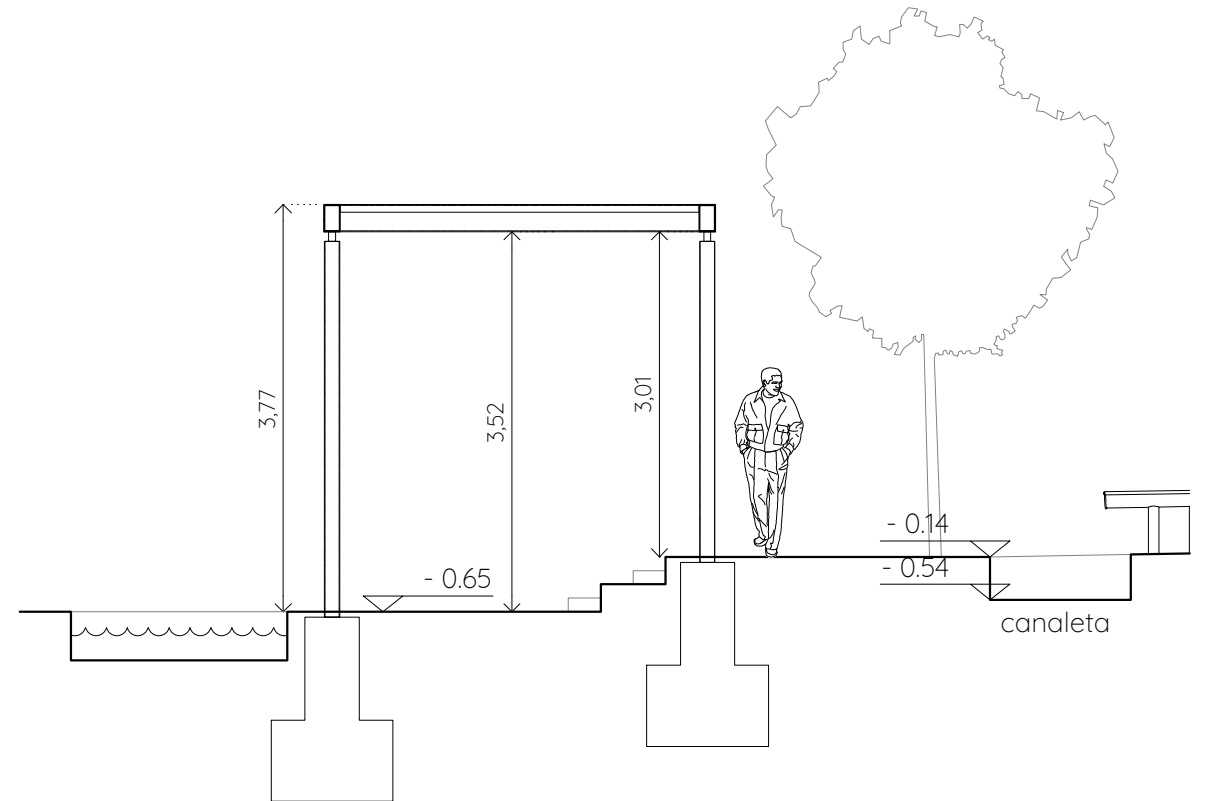
Secció
