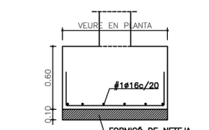
SABATA AÏLLADA
