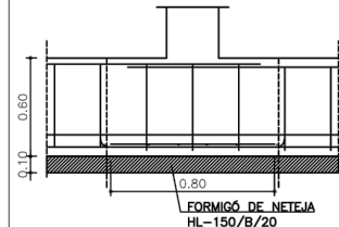
A1_E 1:25 A3_E 1:50
