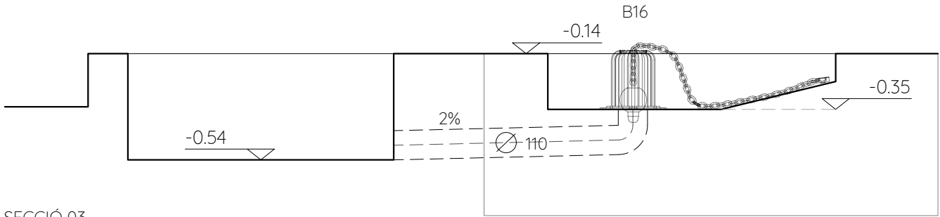
SECCIÓ 03
