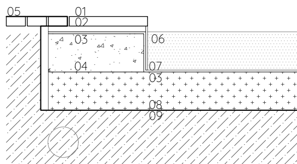
SECCIÓ 01
