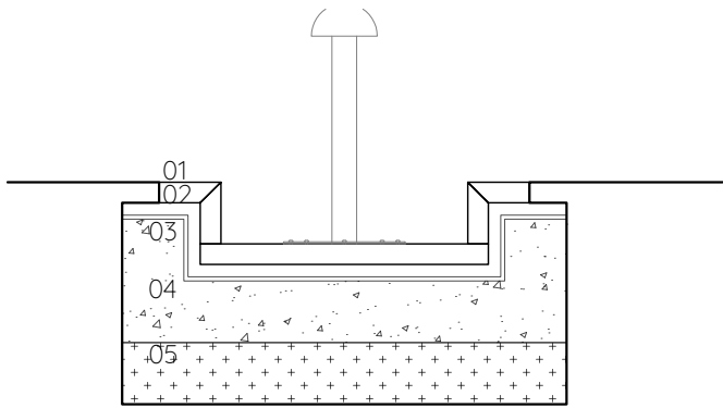
SECCIÓ 02
