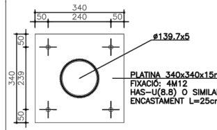
A1_E 1:10 A3_E 1:20
