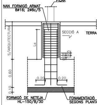
SECCIÓ A
